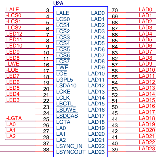
DSP56720_144
