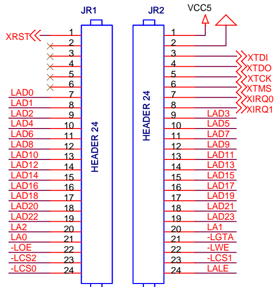
A3P-MRAM module
